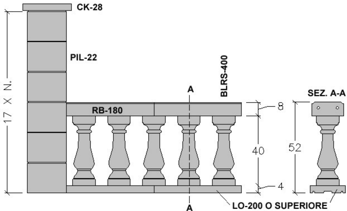
COLONNINA TONDA h 40 CON CORRIMANO RB-180 E ZOCCOLO LO-200 (O SUPERIORE)
