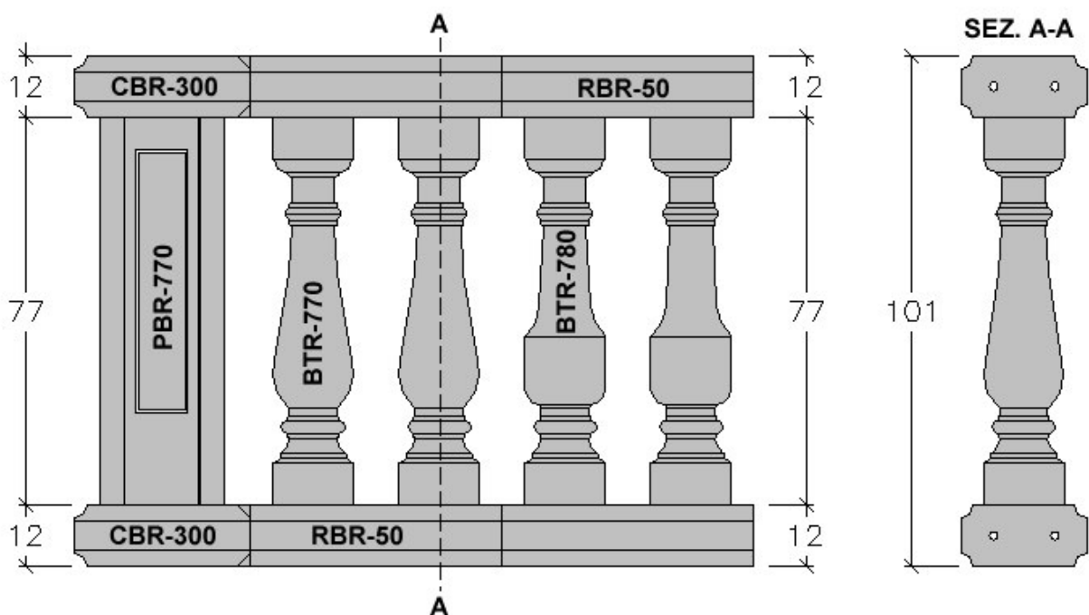
COLONNINA TONDA h 77 CON CORRIMANO E ZOCCOLO RBR-50
